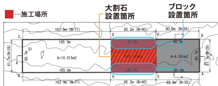
▲ 施工場所の平面図
