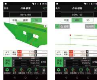
▲3次元測量画面(No.3函渠)
